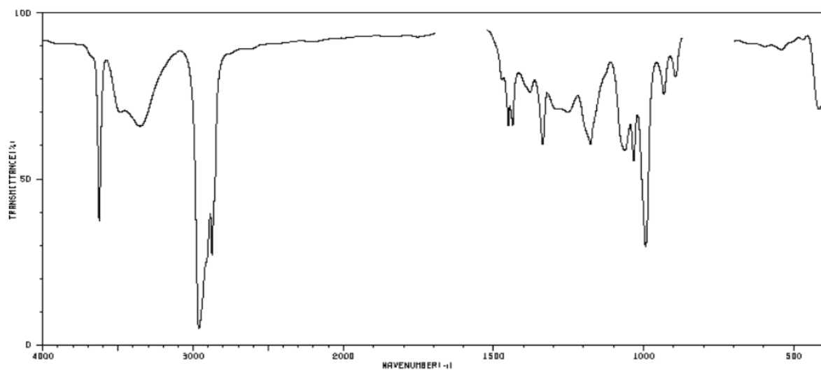
IR-A9 C 4 H 7 OCl
