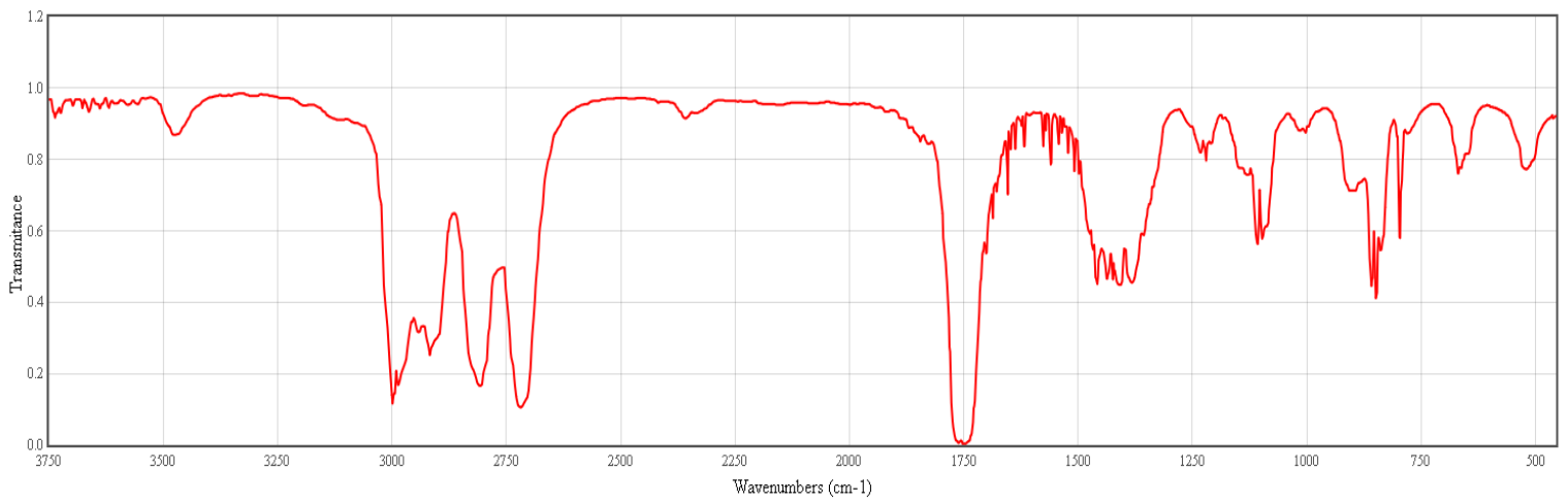
IR-A4 C 3 H 6 O
