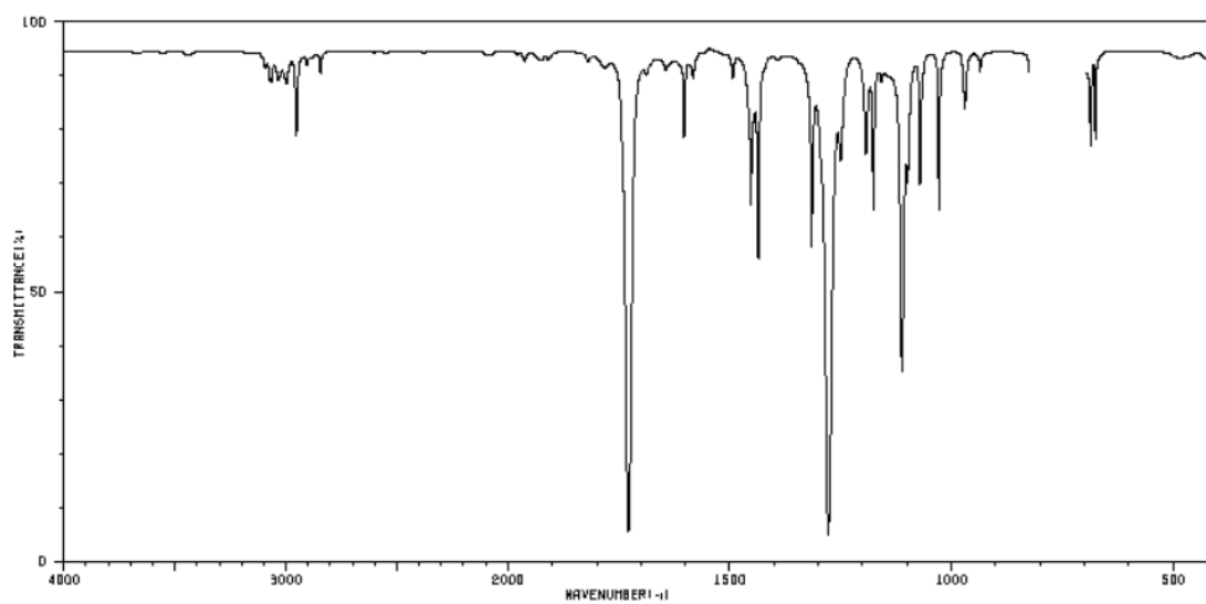
IR-A11 C 8 H 6 N 2 O
