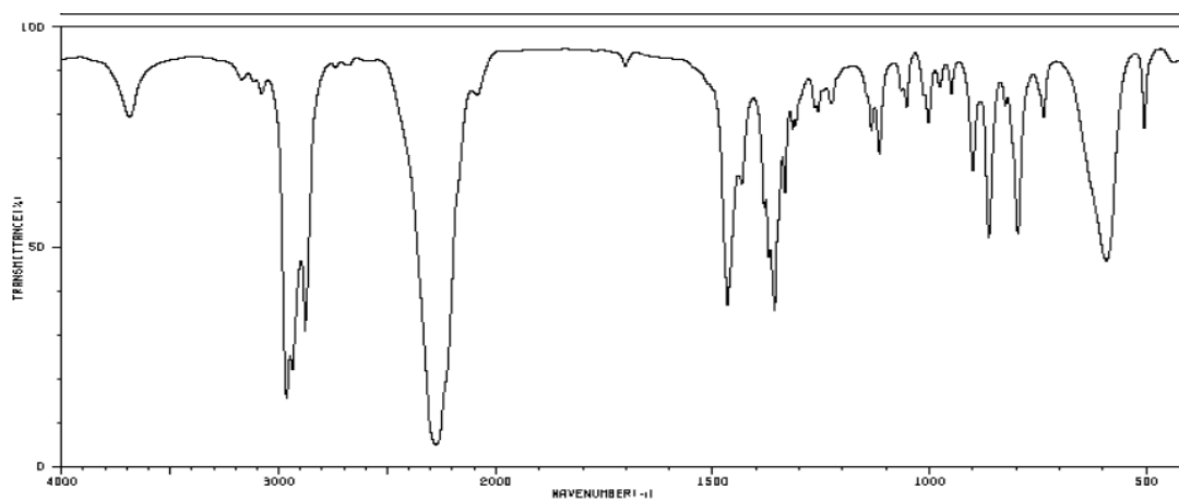
IR-A12 C 5 H 9 NO
