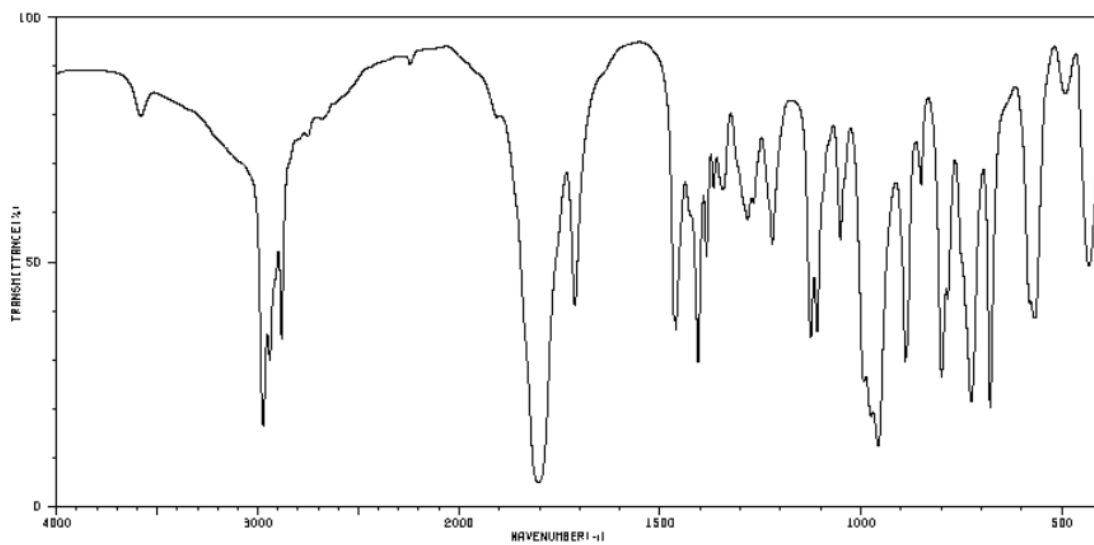
IR-A9 C 4 H 7 OCl
